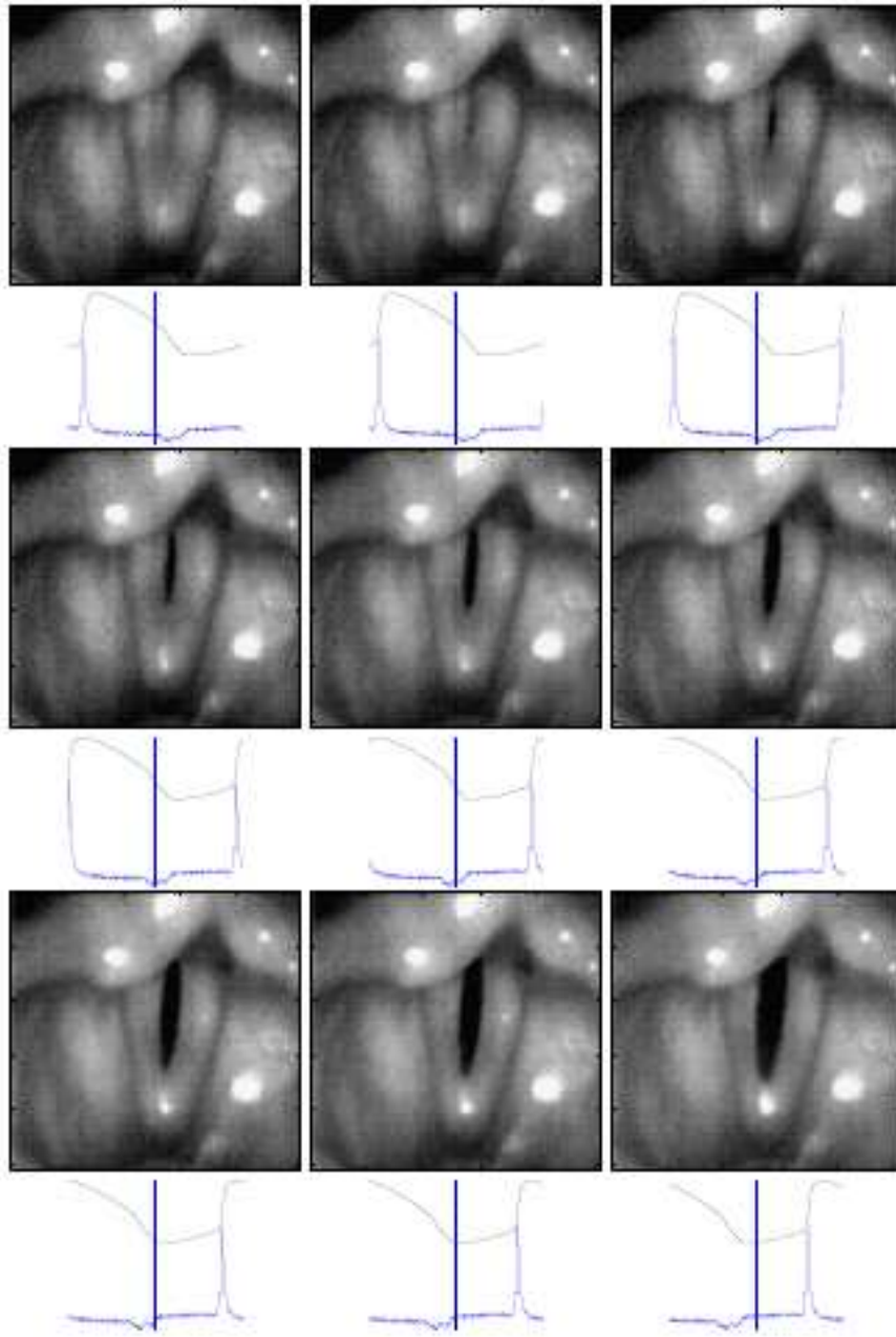
Figura 7.12: Visualização de picos duplos de abertura por cinematografia ultrarrápida e eletroglotografia simultâneas (locutor em fonação normal e frequência fundamental igual a 110 Hz - sinais EGG e DEGG) [10].
