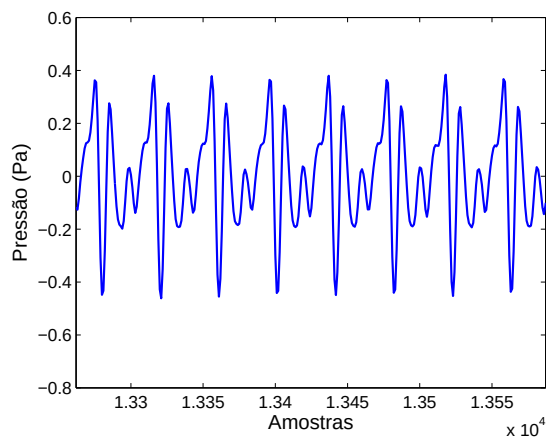
Figura 3.3: Exemplo de um sinal de voz (trecho da vogal sustentada /a/ obtida com uma frequência de amostragem f_s=44.100 Hz).
