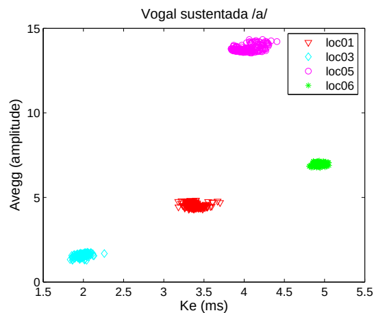
Figura 7.15: Discriminação visual entre os locutores 01, 03, 05 e 06, utilizando a vogal sustentada /a/
